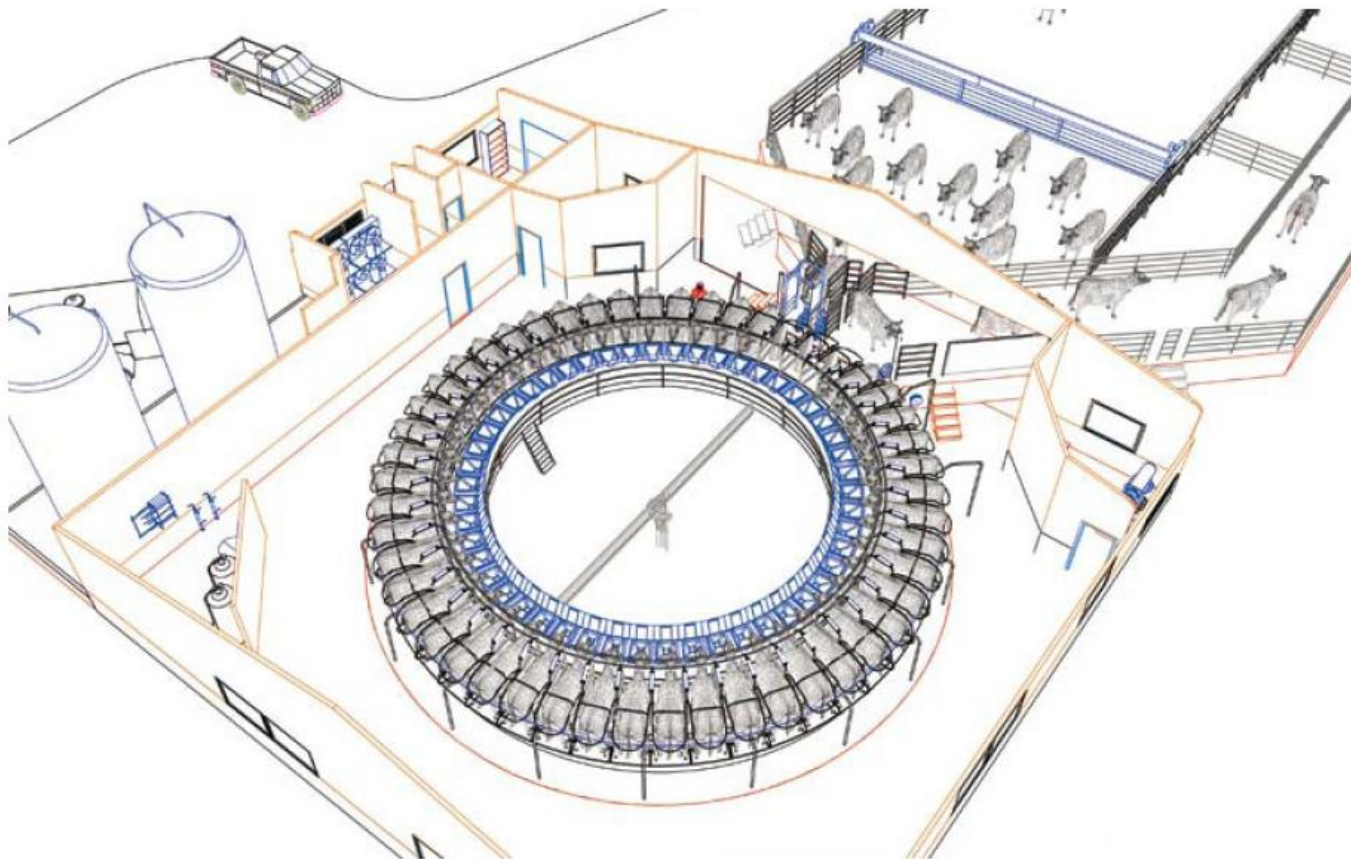
Rotativa Paralela
